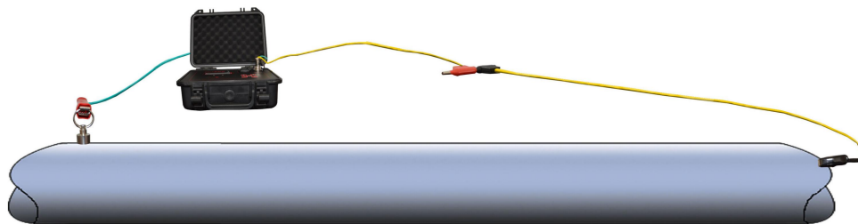
图6 回路法接线示意图
