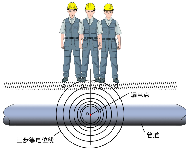
图16 三步等电位示意图
