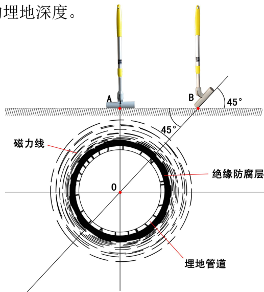
图10 管道45° 法测深图
