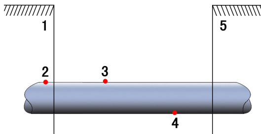
图17 管道防腐层破损处开挖验证示意图
