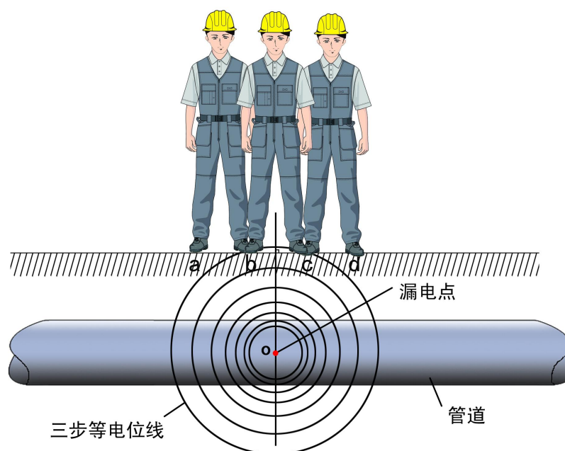
图16 三步等电位示意图
