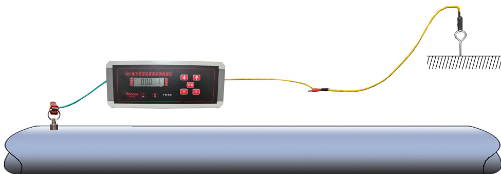
图4 单边接地示意图
