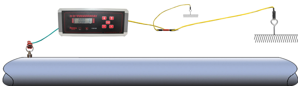
图6 回路法接线示意图
