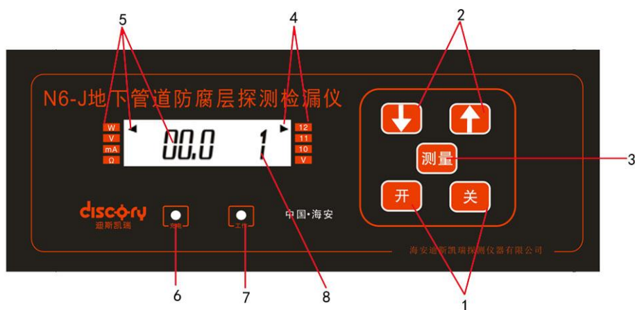
图 1 发射机前面板示意图
