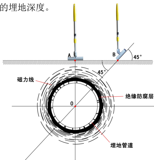
图10 管道45° 法测深图
