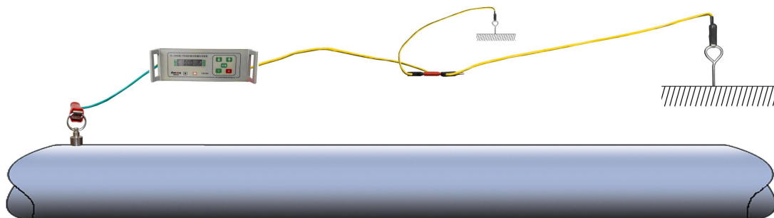
图7 远接地回路示意图
