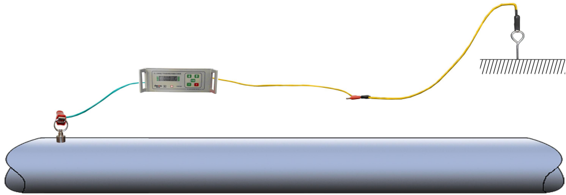
图4 单边接地示意图
