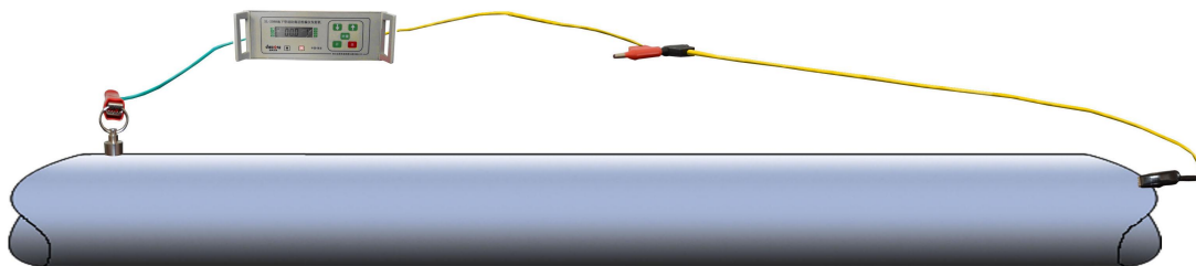
图6 回路法接线示意图
