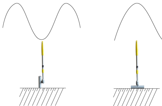
图8 零值法探测示意图
