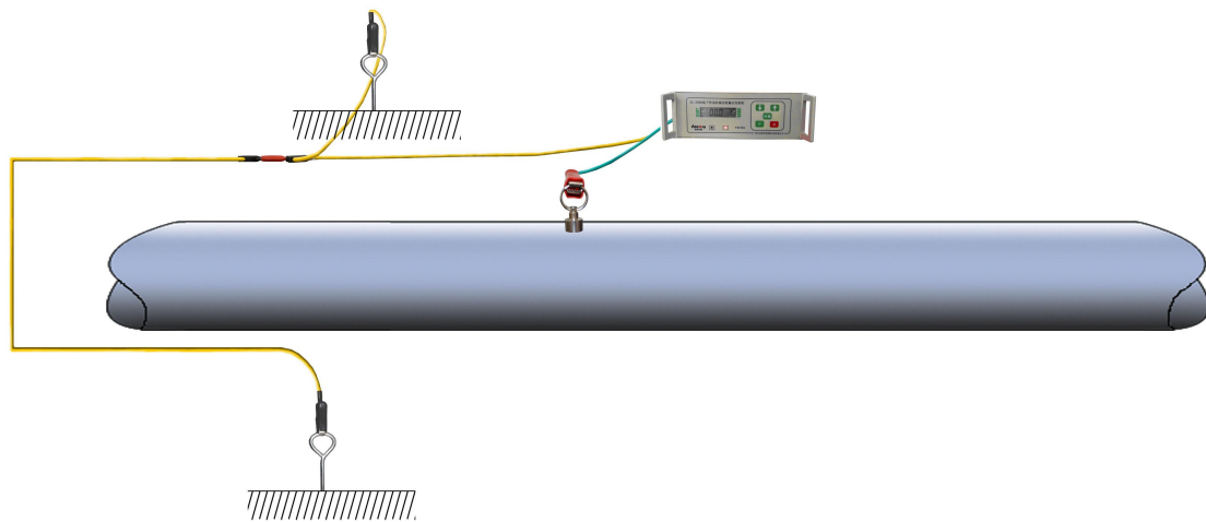
图5 双边接地示意图
