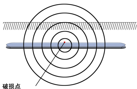
图11 地下破损点电位梯度立面分布图
