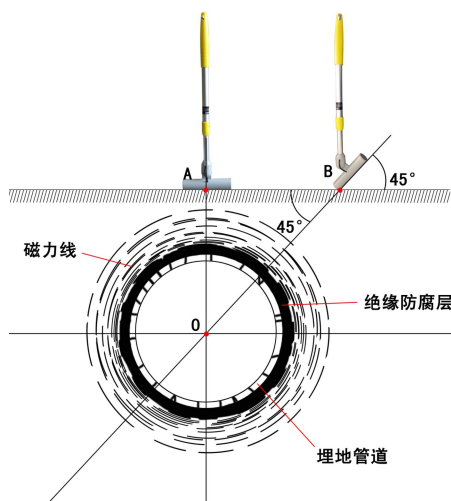
图10 管道 45^\circ 法测深图
